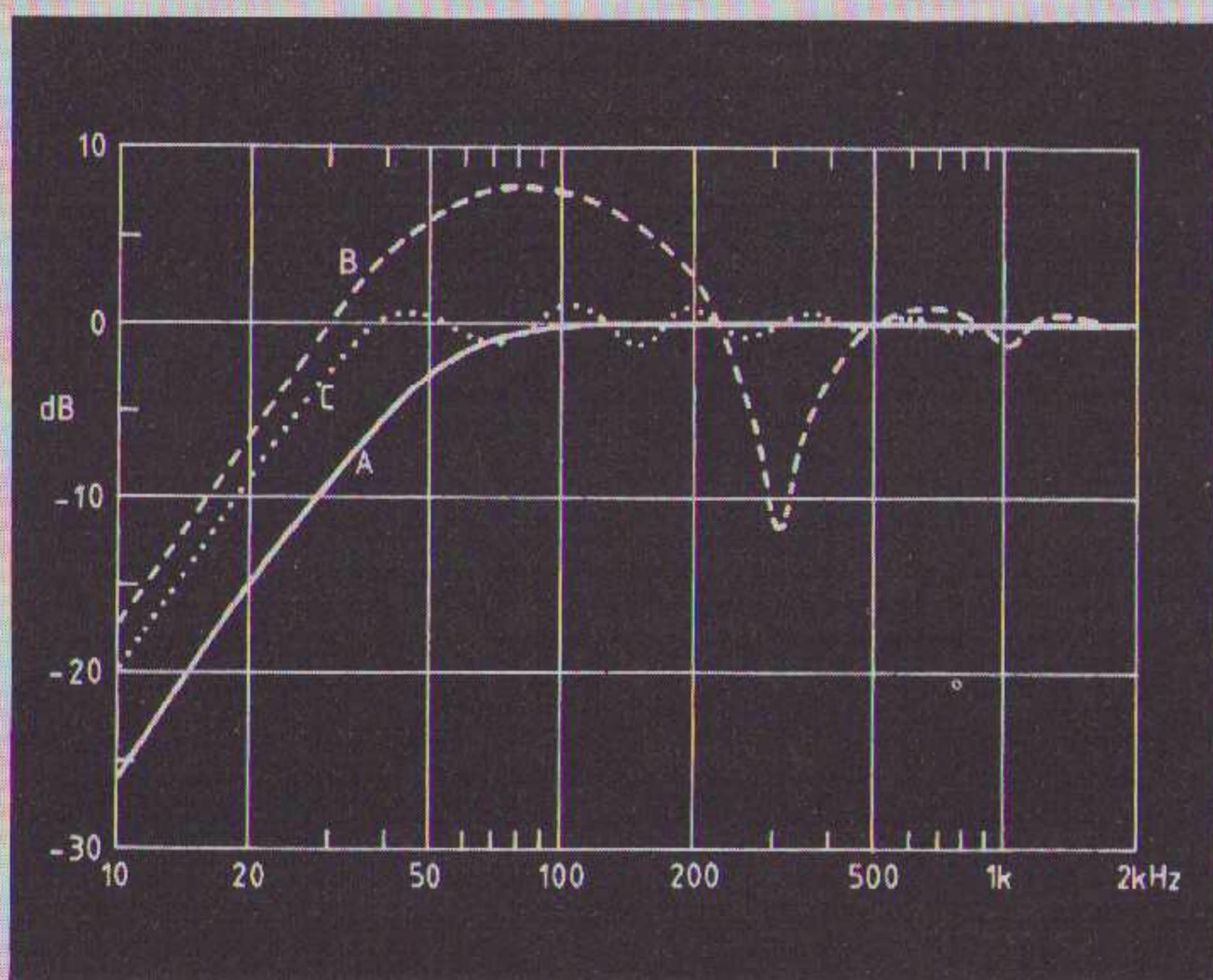
Fig. 45. Vermogensresponsie van een gesloten box met q = 0,7 en resonantiefrequentie van 50 Hz.
